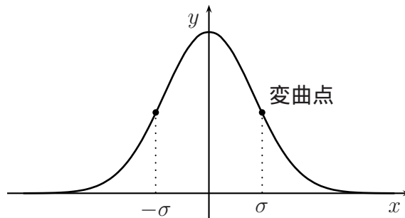
図 2.1: 正規分布のグラフ
